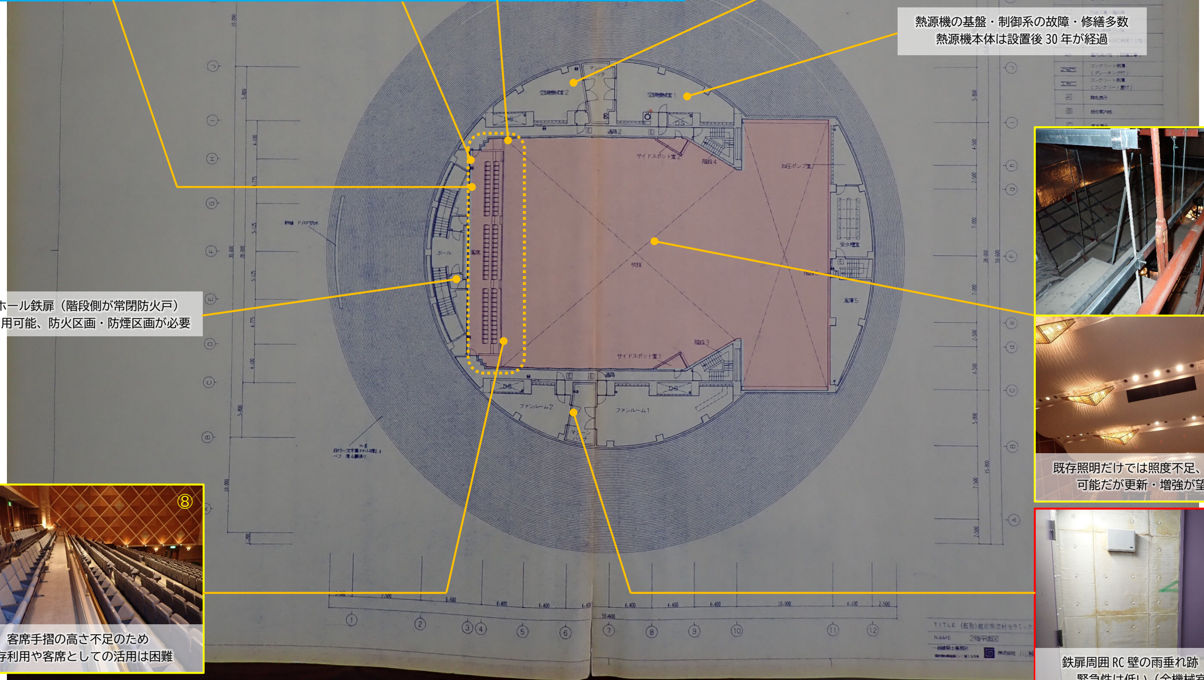
客席後方部の仕上材に有孔吸音板が使用されており、客席前方部に比べて反響音が少ない
